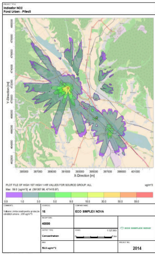
Figura nr. 3-16 Creștere nivel Fond urban Aglomerarea Pitești – industrie – indicator NO2, medie orară
