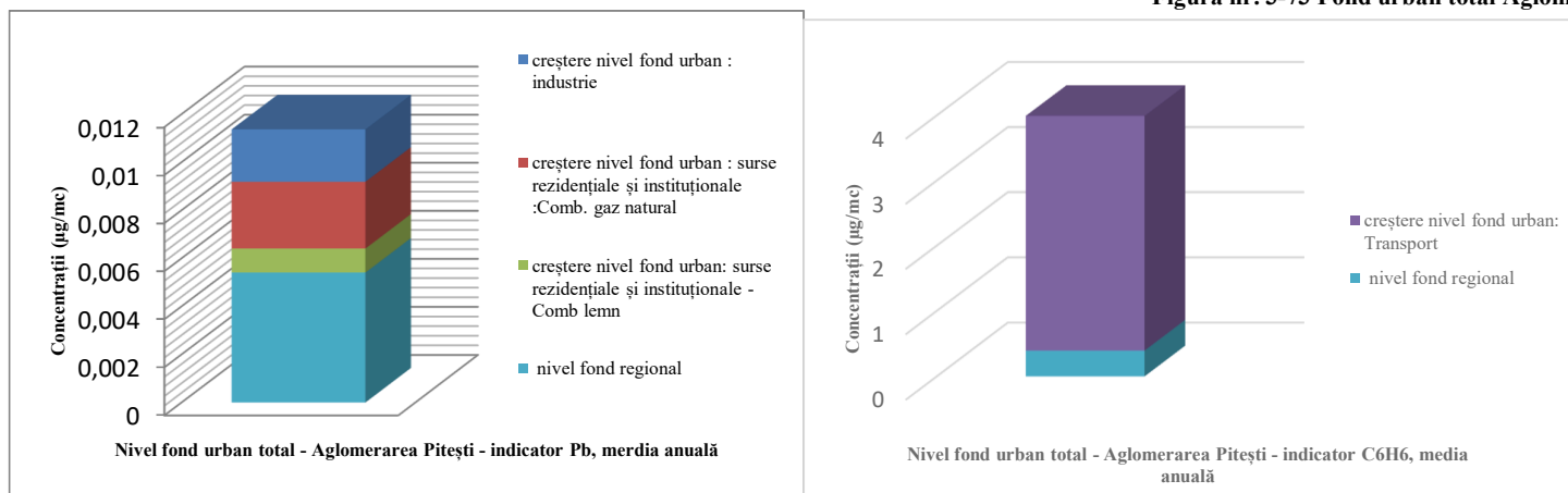
Figura nr. 3-74 Fond urban total Aglomerarea Pitești – indicator Pb
