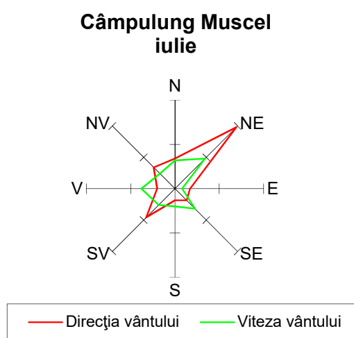
Figura nr. 3-145 Roza vânturilor lunară
