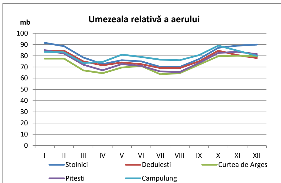
Figura nr. 2-28 Umezeala relativă a aerului – anul 2014
