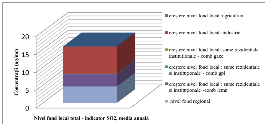
Figura nr. 3-130 Fond local total zona Argeș - indicator SO 2
