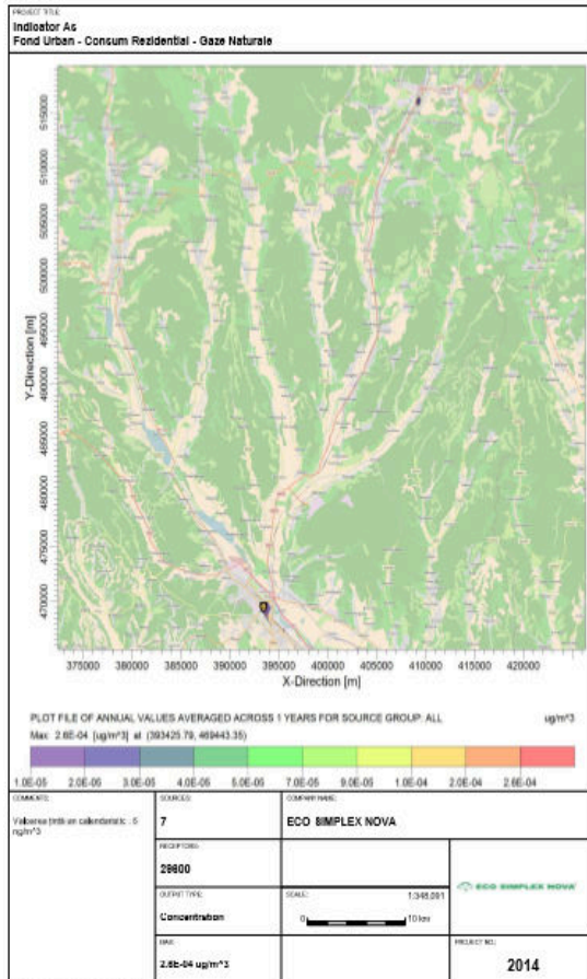
Figura nr. 3-31 Creștere nivelFond urban zona Argeș - consum rezidențial GN – indicator As, medie anuală
