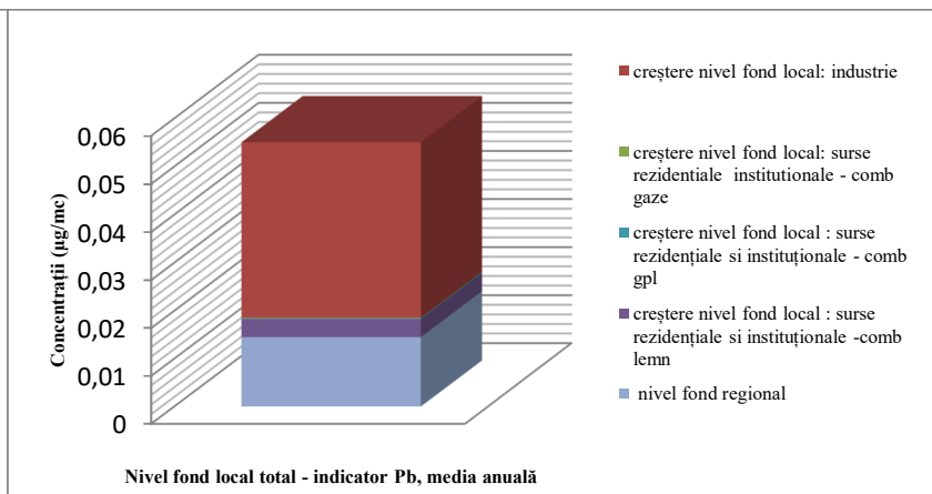
Figura nr. 3-139 Fond local total zona Argeș – indicator Pb
