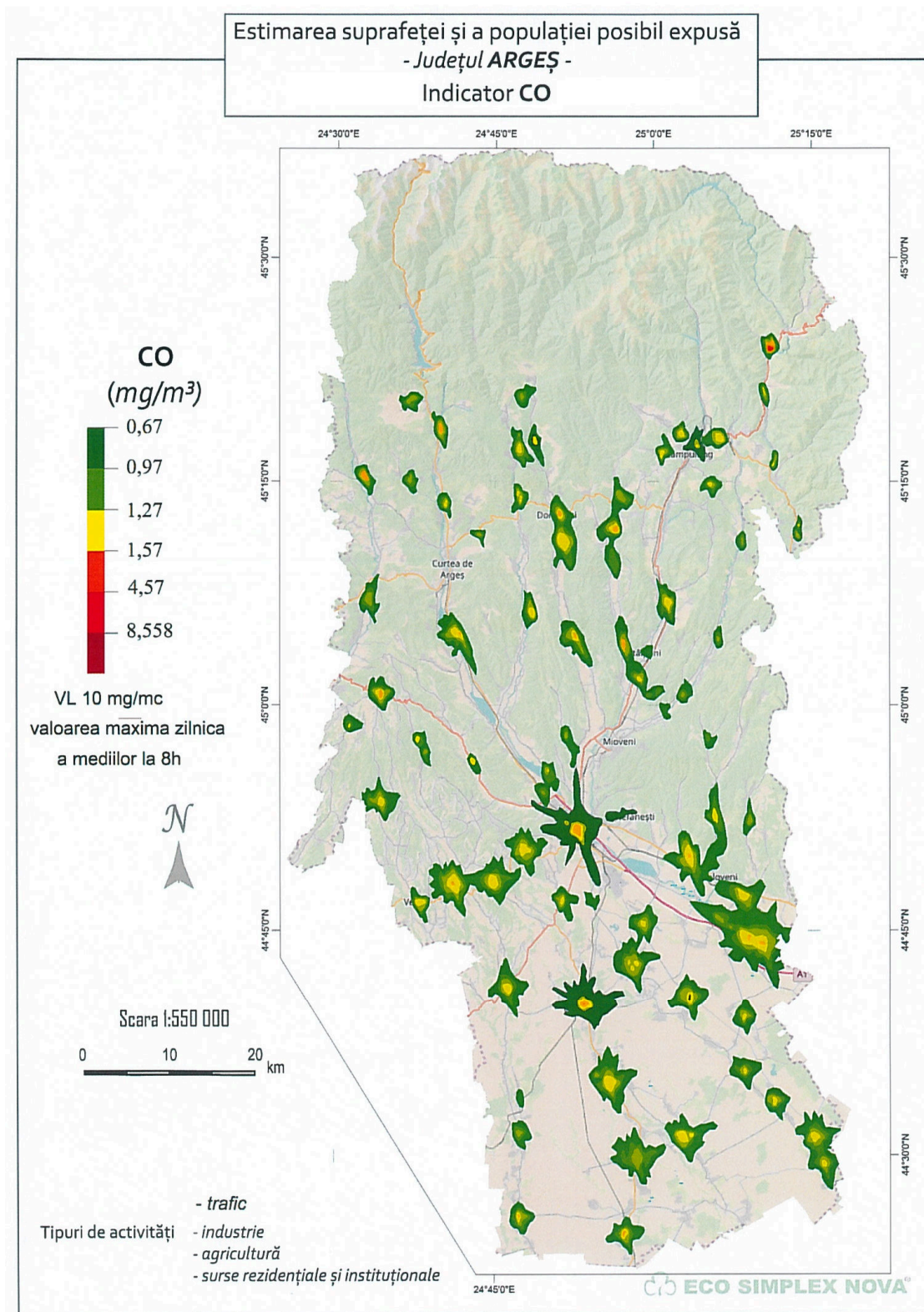
Figura nr. 2-14 Harta – Estimarea suprafeței zonei și a populației posibil expusă poluării – indicator CO Sursa: harta prelucrată cu programul ARC GIS versiunea 10.3 de modificat harta
