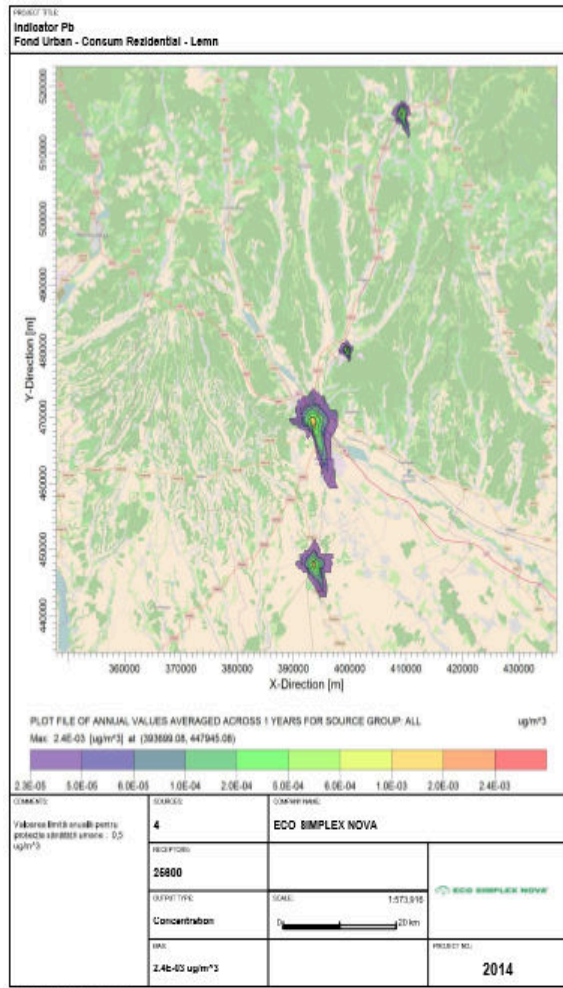
Figura nr. 3-52 Creștere nivel Fond urban zona Argeș - consum rezidențial lemn – indicator Pb, media anuală
