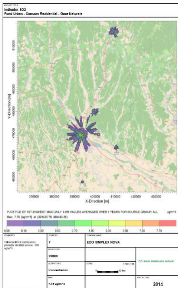
Figura nr. 3-25 Creștere nivelFond urban zona Argeș - consum rezidențial GN- indicator SO2, medie orară
