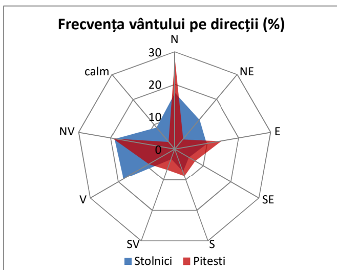
Figura nr. 2-33 Frecvența vântului – anul 2014
