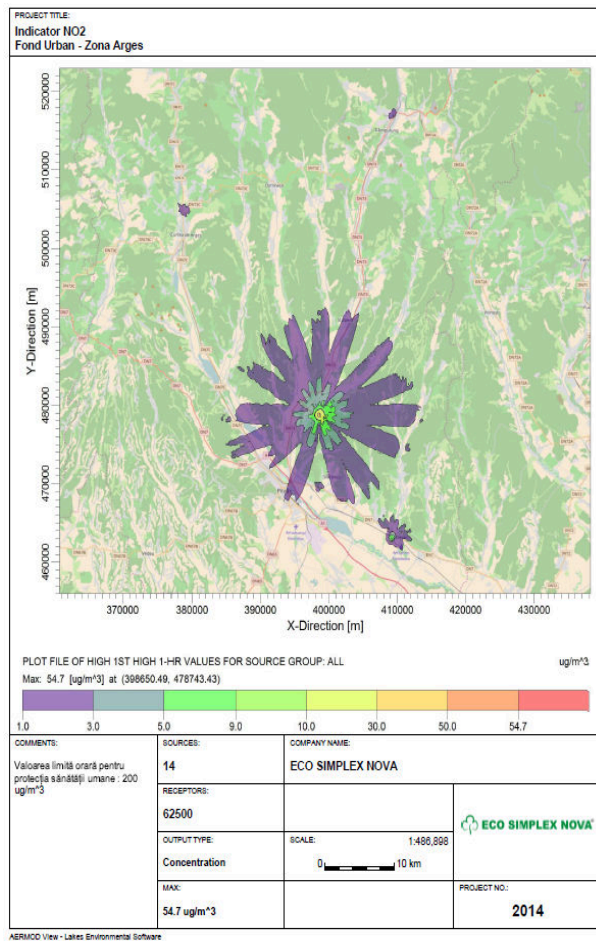
Figura nr. 3-4 Creștere nivel Fond urban zona Arges - industrie - indicator NO2 – media orară
