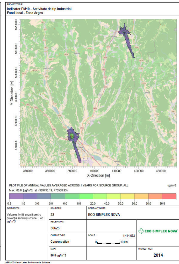
Figura nr. 3-80 Creștere nivelFond local – industrie – indicator CO, medie la 8h
