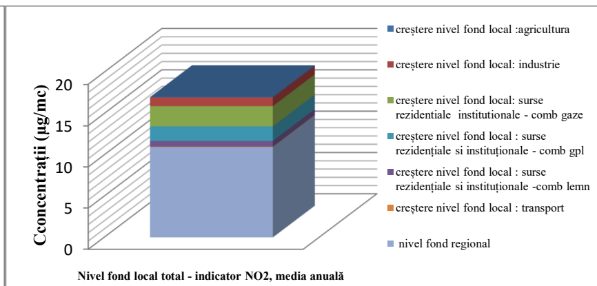
Figura nr. 3-131 Fond local total zona Argeș – indicator NO 2
