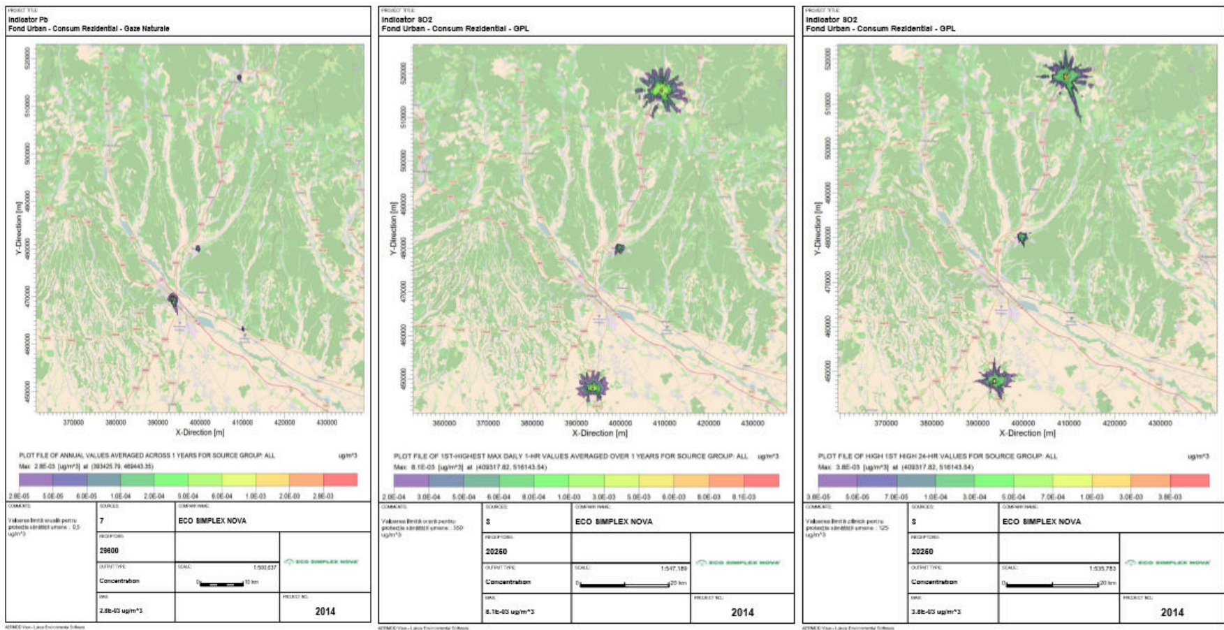
Figura nr. 3-34 Creștere nivelFond urban zona Argeș - consum rezidențial GN- indicator Pb, medie anuală
