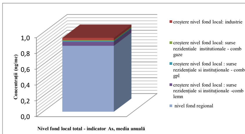
Figura nr. 3-136 Fond local total zona Argeș - indicator As
