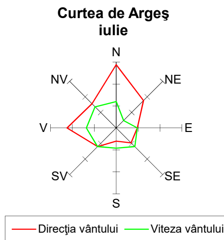
Figura nr. 3-146 Roza vânturilor lunară
