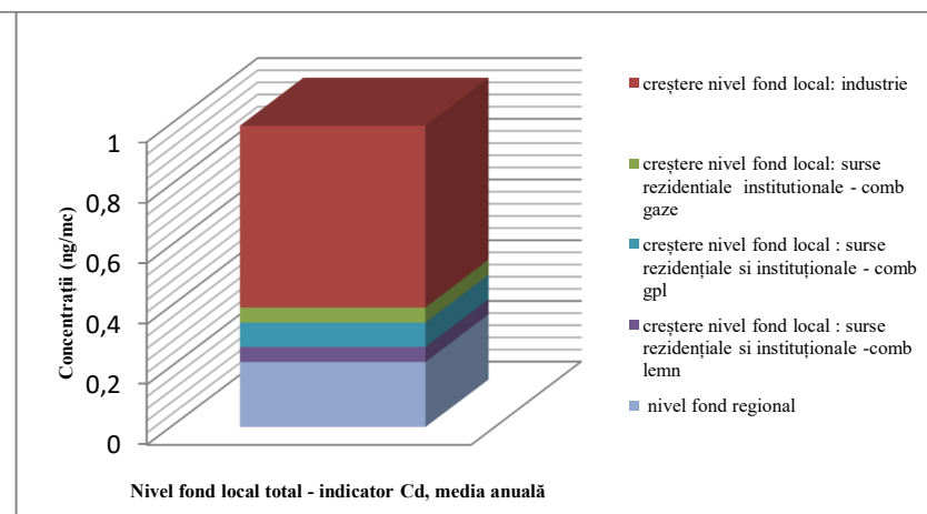
Figura nr. 3-137Fond local total zona Argeș - indicator Cd
