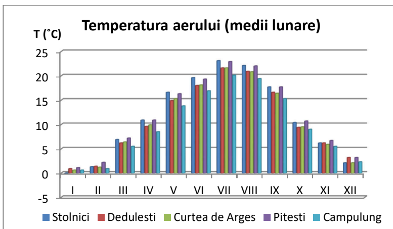
Figura nr. 2-27 Medii lunare ale temperaturii măsurate la stațiile meteo – anul 2014
