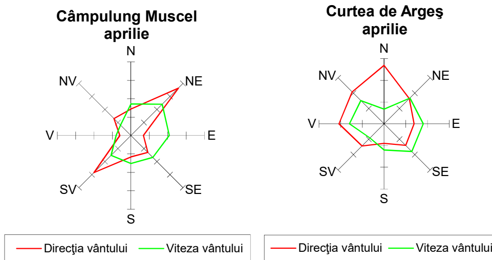
Figura nr. 3-143 Roza vânturilor lunară
