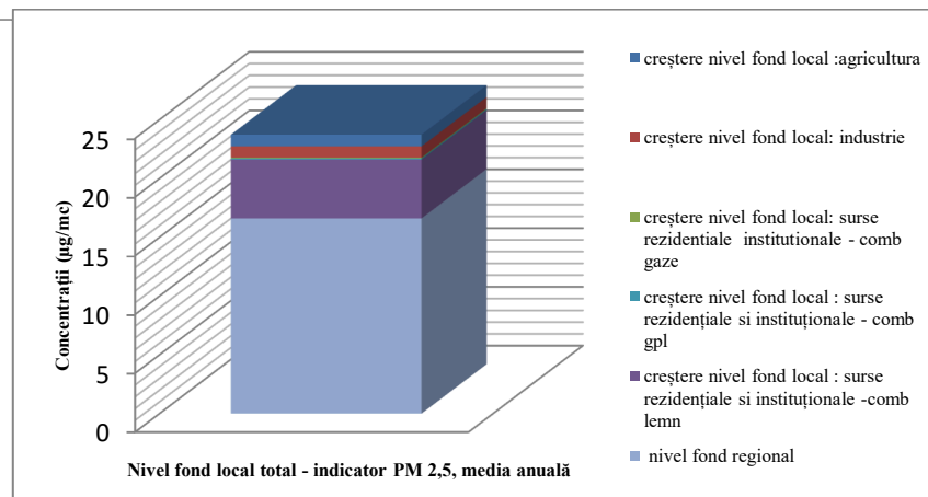
Figura nr. 3-135 Fond local total zona Argeș - indicator PM2,5
