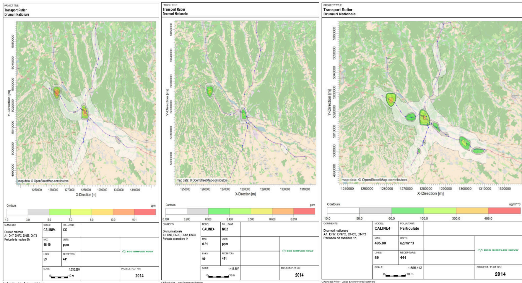
Figura nr. 3-127 Creștere nivel Fond Transport rutier – indicator CO
