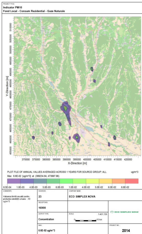
Figura nr. 3-100 Creșterea nivel Fond local – consum rezidențial GN- indicator PM10, media anuală
