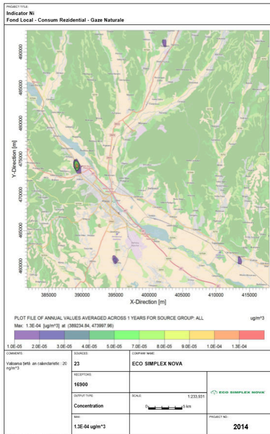
Figura nr. 3-103 Creștere nivel Fond local – consum rezidențial GN – indicator Ni, media anuală
