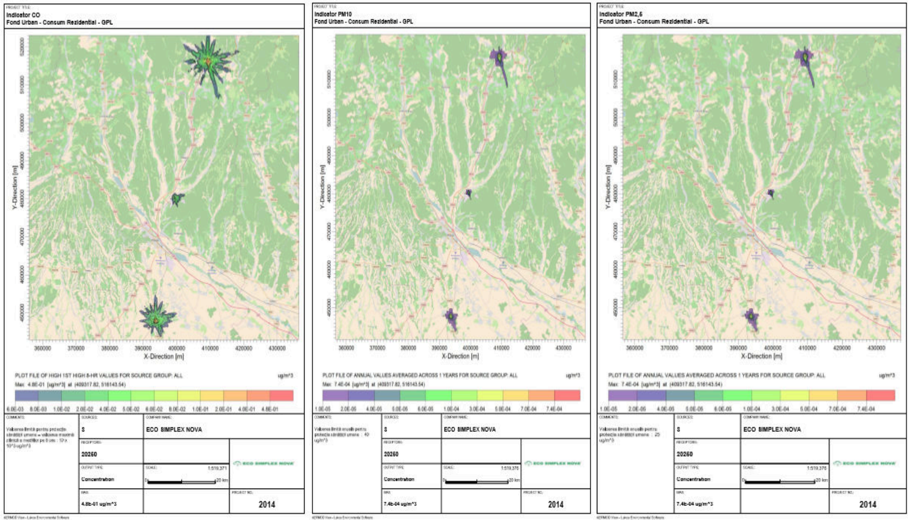
Figura nr. 3-40 Creștere nivel Fond urban zona Argeș - consum rezidențial GPL – indicator CO, val max. zilnică a mediilor la 8 ore
