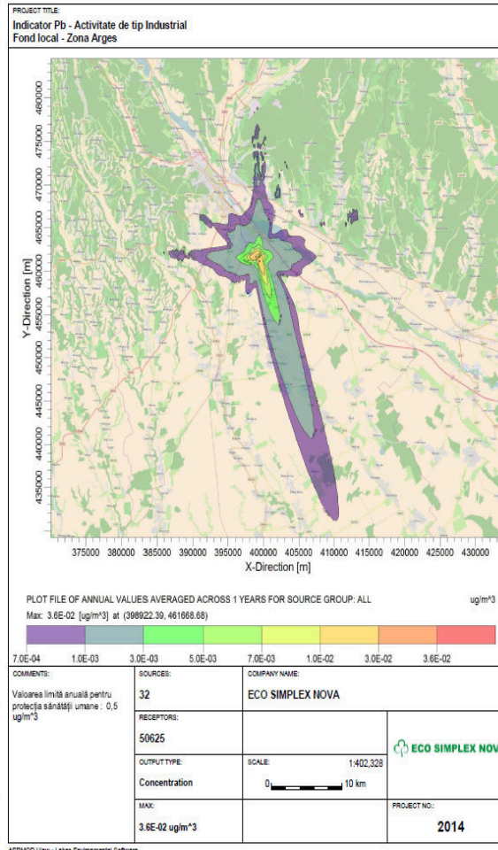
Figura nr. 3-86 Creștere nivel Fond local – industrie – indicator Pb, medie anuală
