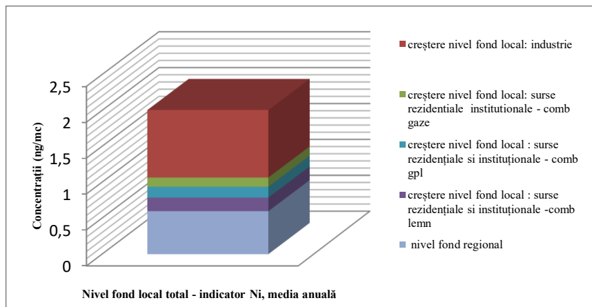
Figura nr. 3-138 Fond local total zona Argeș - indicator Ni
