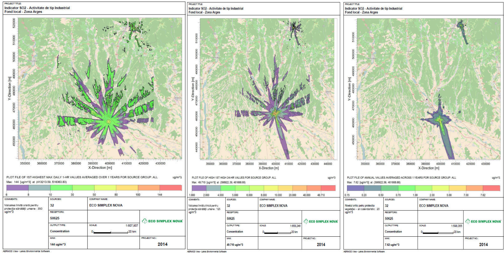
Figura nr. 3-76 Creștere nivelFond local – industrie – indicator SO 2- media orară
