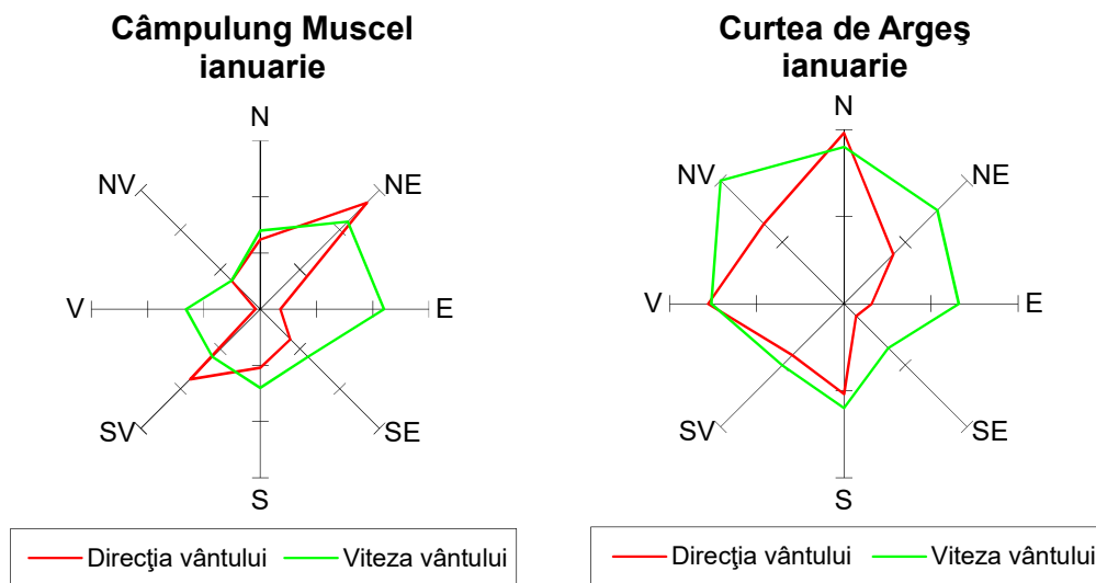
Figura nr. 3-141 Roza vânturilor lunară
