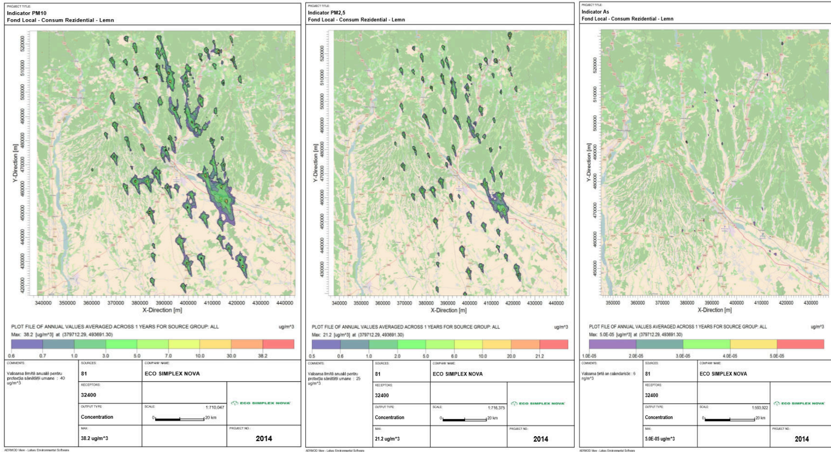
Figura nr. 3-121 Creștere nivel Fond local – consum rezidențial lemn- indicator PM10, media anuală
